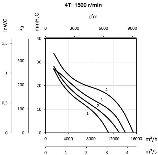
1 : HCH-56-4T-0.75 2 : HCH-56-4T-1
