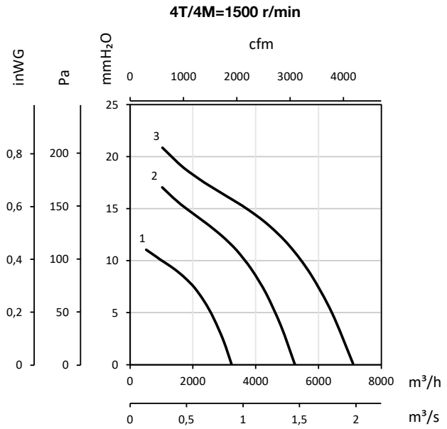
1 : HCH-35-4T 2 : HCH-40-4T-0.33
