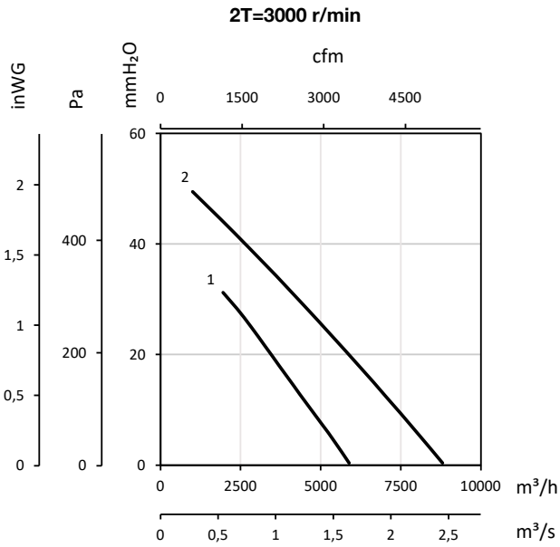
1 : HCH-35-2T 2 : HCH-40-2T-1.5
